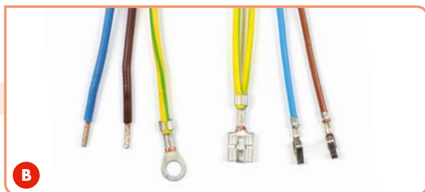
B Finiture particolari lato opposto alla spina, morsettiere, passacavi, blocchetti, commerciali o su disegno del Cliente.
